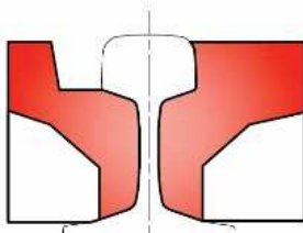
WERSJA 2 - "ETP" szyny: 49E1 (S49); płyta CBP rozstaw 670 mm
