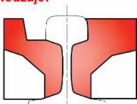
WERSJA 1 - "CBP" szyny: 49E1 (S49); płyta CBP rozstaw 600 mm
